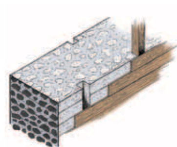
I. Opus caementicium
