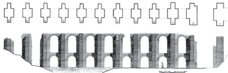
Κάτοψη και όψη της νότιας πεσσοστοιχίας (γέφυρας) στις πηγές του Αγίου Γεωργίου
