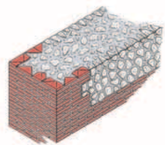
VI. Opus mixtum
