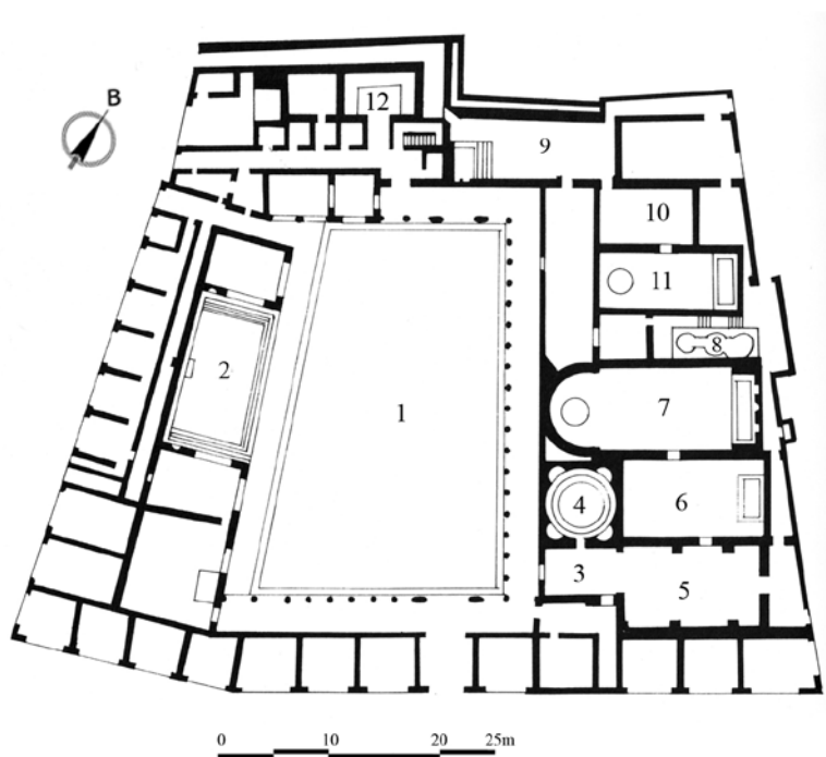
Σταβιανές θέρμες της Πομπηίας, κάτοψη
