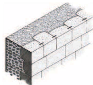
II. Opus quadratum
