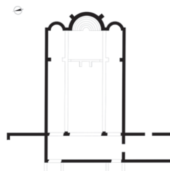
Κάτοψη της Βασιλικής Γ
