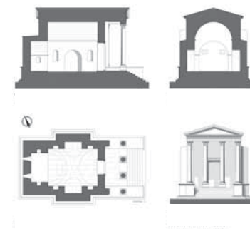
Το ναόσχημο Μαυσωλείο 2 και η γραφική του αναπαράσταση
