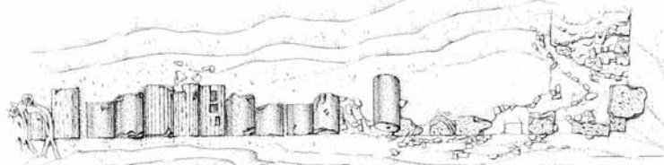
Τοίχος με σπόδια ανάμεσα στους πεσσούς του Υδραγωγείου στο ΝΔ σκέλος του τείχους
